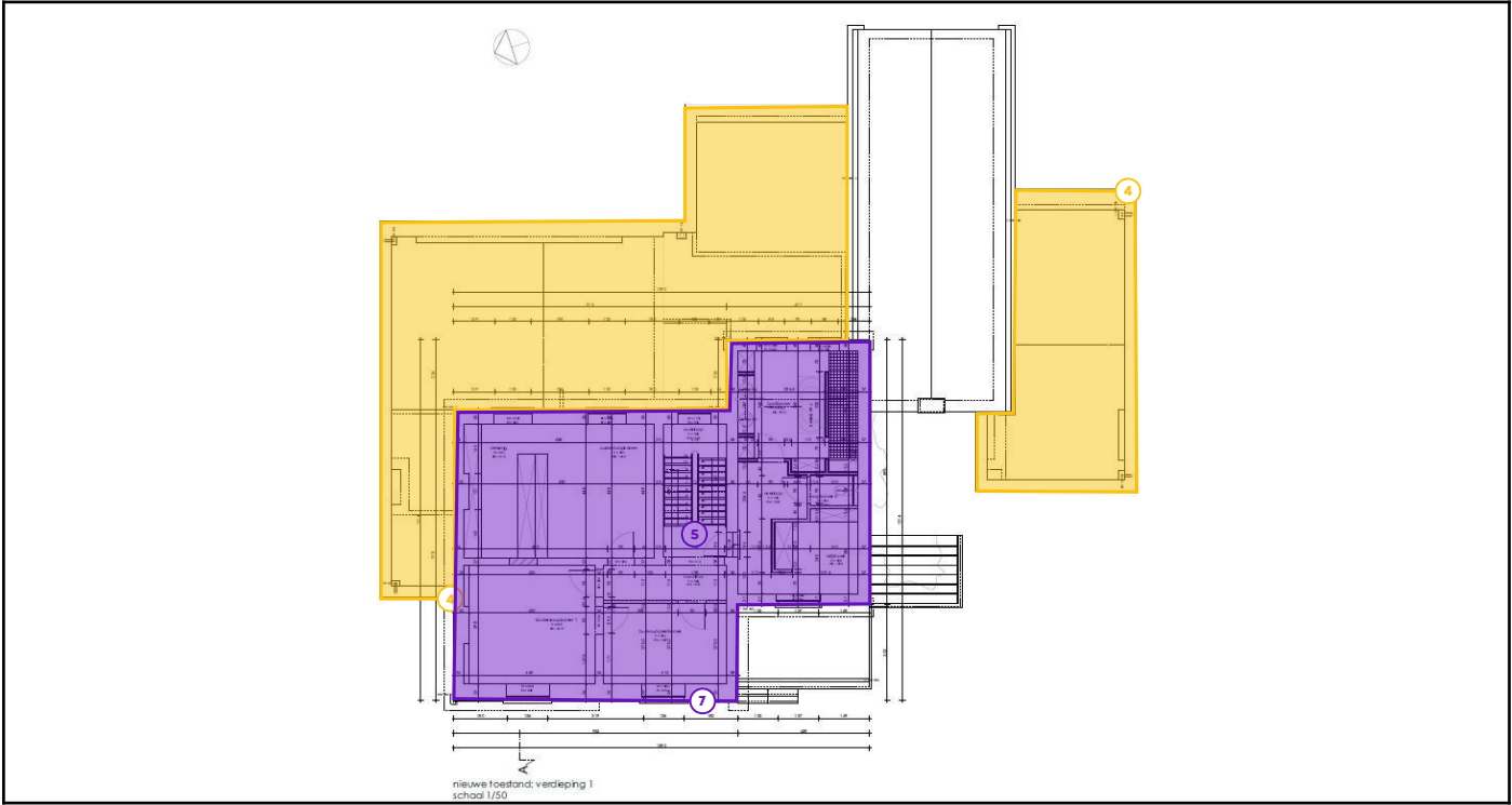
Legende van plan 1.7: HOOFDGEBOUW verdiep +1 plafonds
