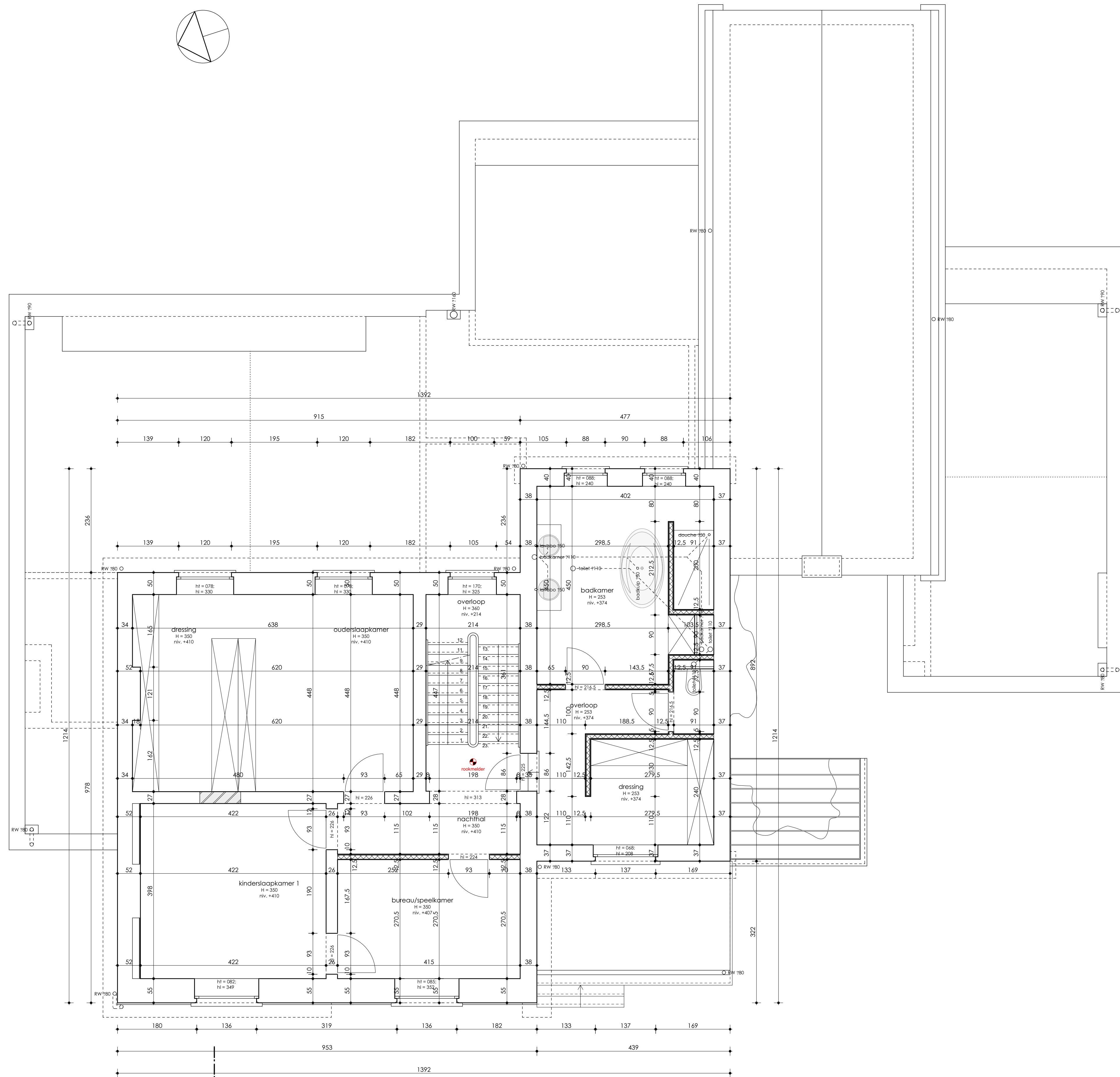
nieuwe toestand: verdieping 1 schaal 1/50
